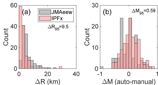
図 1: 震源位置の誤差とマグニチュードの誤差
